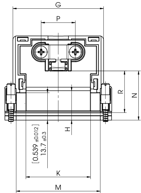
view of the hood without lid Ansicht der Haube ohne Deckelseite
