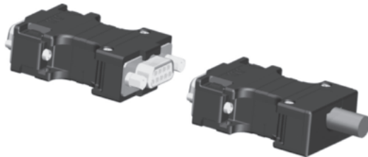
Plastic hoods FAH with straight cable outlet in shell size 1, cable to cable connection. Kunststoffhauben FAH mit geradem Kabelausgang in der Gehäusegröße 1, fliegende Verbindung.
