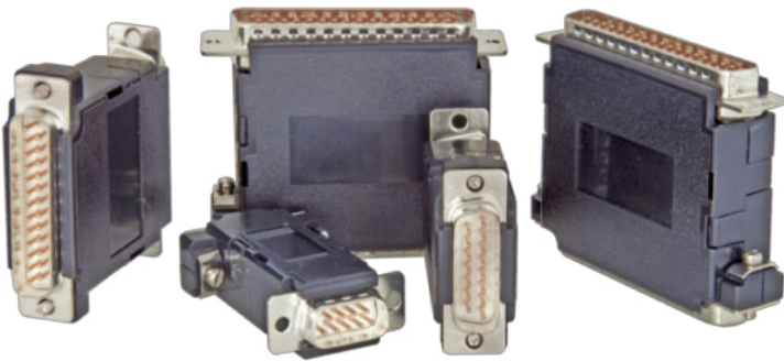
Plastic adapter hoods series F1069 in shell sizes 1 - 5 (with a second connector converts to an adaptor). Kunststoffadapterhaube der Serie F1069 in den Gehäusegrößen 1 - 5 (mit zweitem Steckverbinder als Adapter verwendbar).
